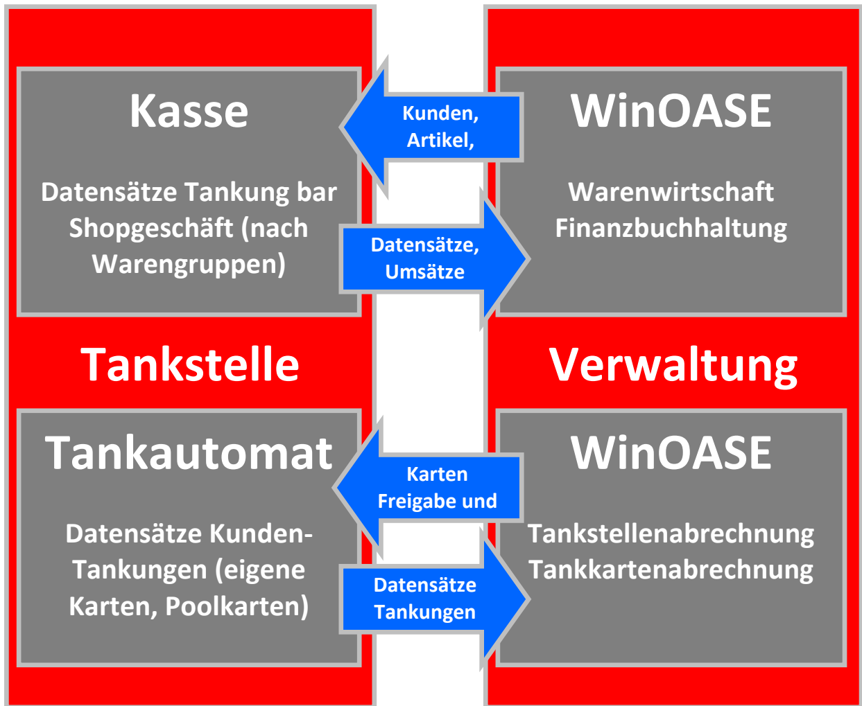
Bild 8 : Datenübertragungen im Tankstellen-Management zwischen Tankstelle (Tankautomat) und verwaltung (WinOASE System)
